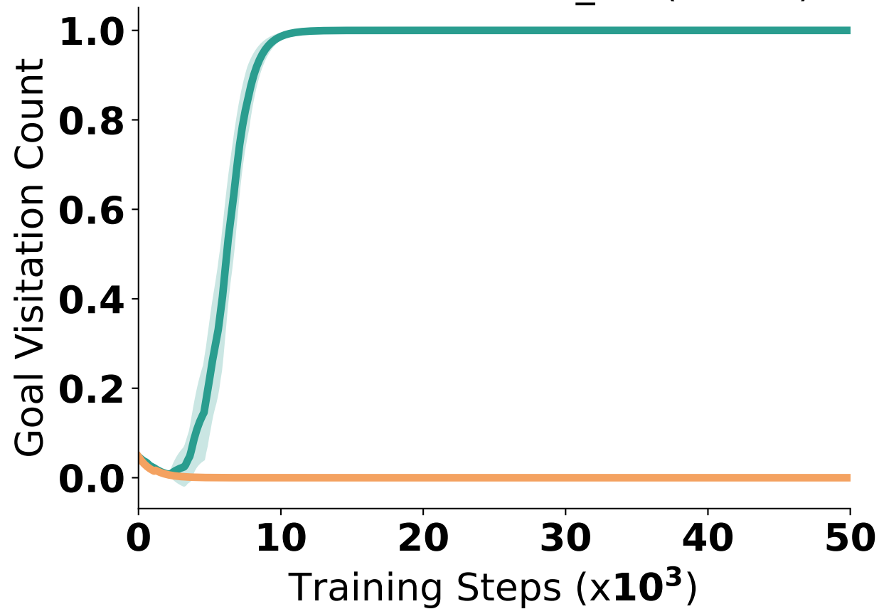
Gridworld-Bottleneck_Ask(20.0%)
